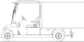
Kompozit Kapalı Kasa E: 1320 x B: 1800 x Y: 1310
