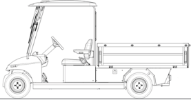
Kasa Örtüsü E: 1310 x B: 1800 x Y: 440
